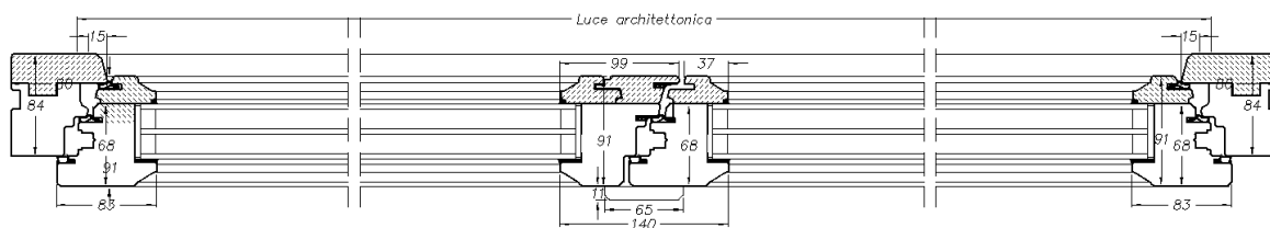
Sezione B-B'
